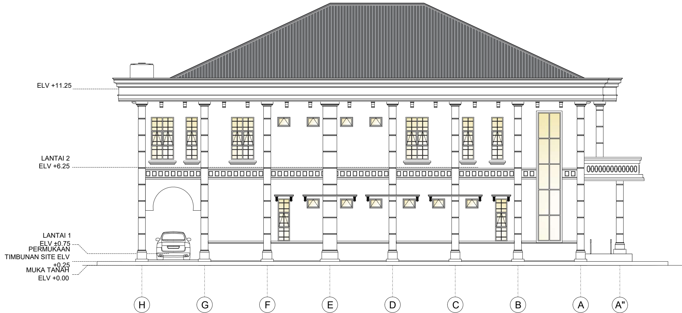
RENCANA TAMPAK SAMPING KIRI SKALA 1 : 150
